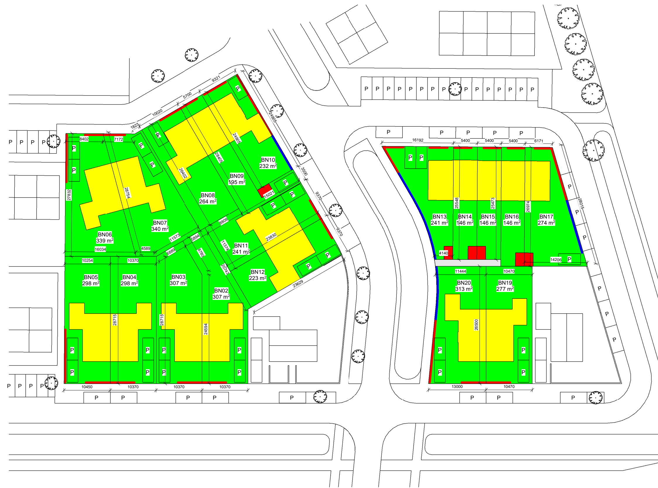
Situatie - totaal Schaal: 1 : 500
